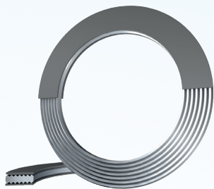
KAMMPROFILDICHTUNG FÜR FLANSCH MIT NUT UND FEDER
