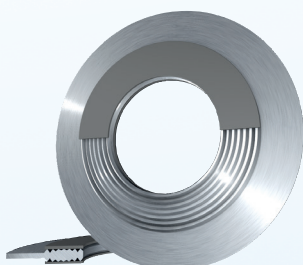
BALLIGE KAMMPROFILDICHTUNG MIT WEICH- STOFFAUFLAGE UND ZENTRIERRING
