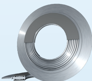
BALLIGE KAMMPROFILDICHTUNG MIT WEICH- STOFFAUFLAGE UND LOSEM ZENTRIERRING
