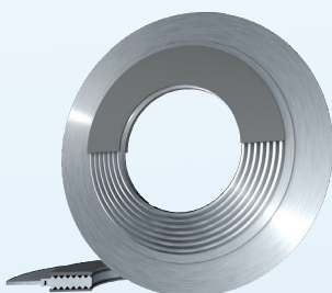
KAMMPROFILDICHTUNG MIT WEICHSTOFF- AUFLAGE UND LOSEM ZENTRIERRING
